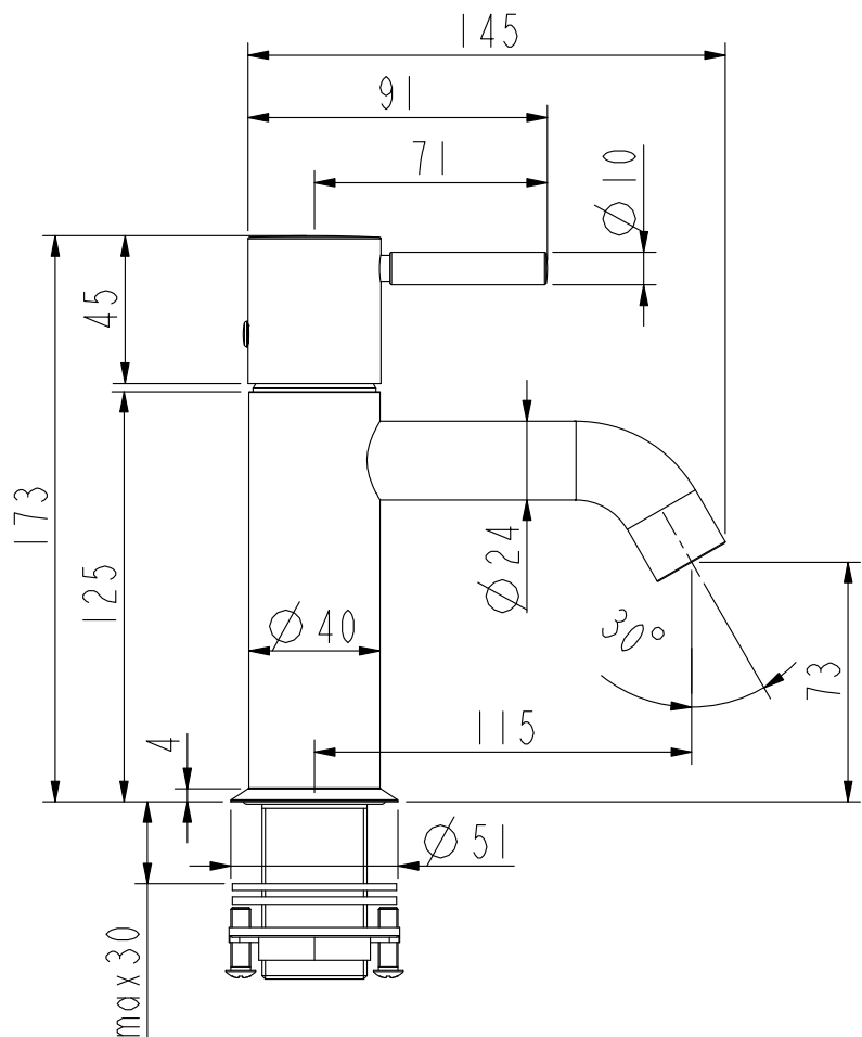
ГАБАРИТНЫЕ РАЗМЕРЫ
