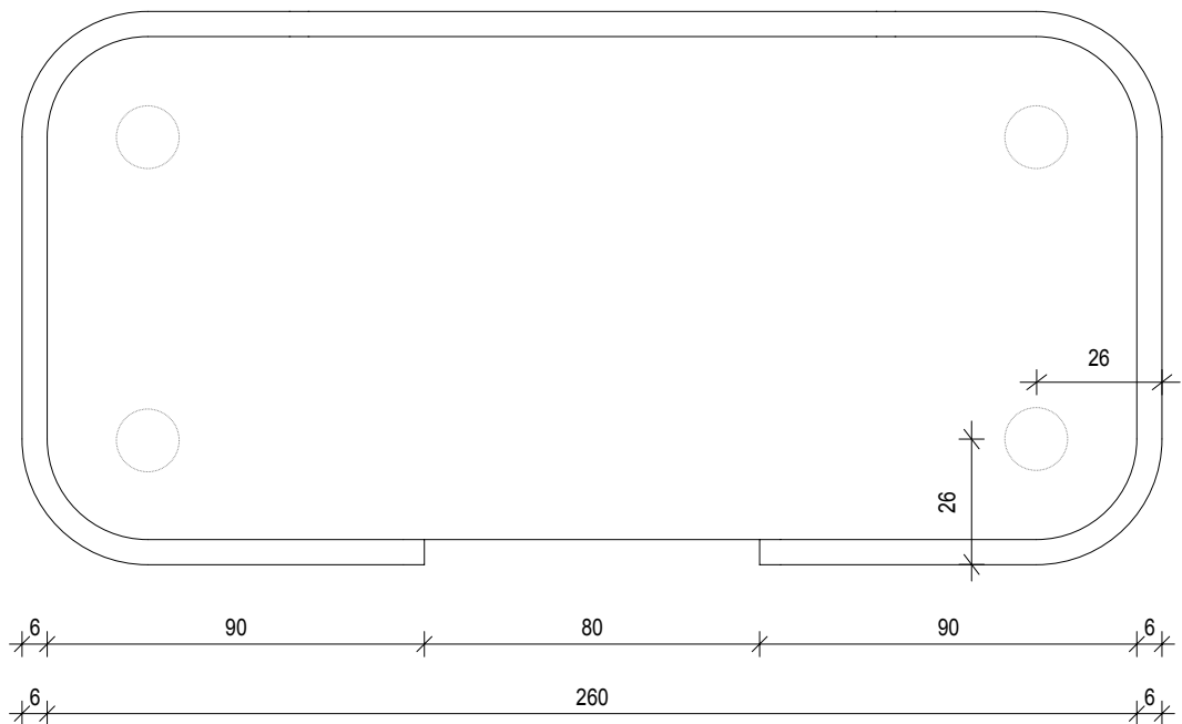
Draufsicht Top view
