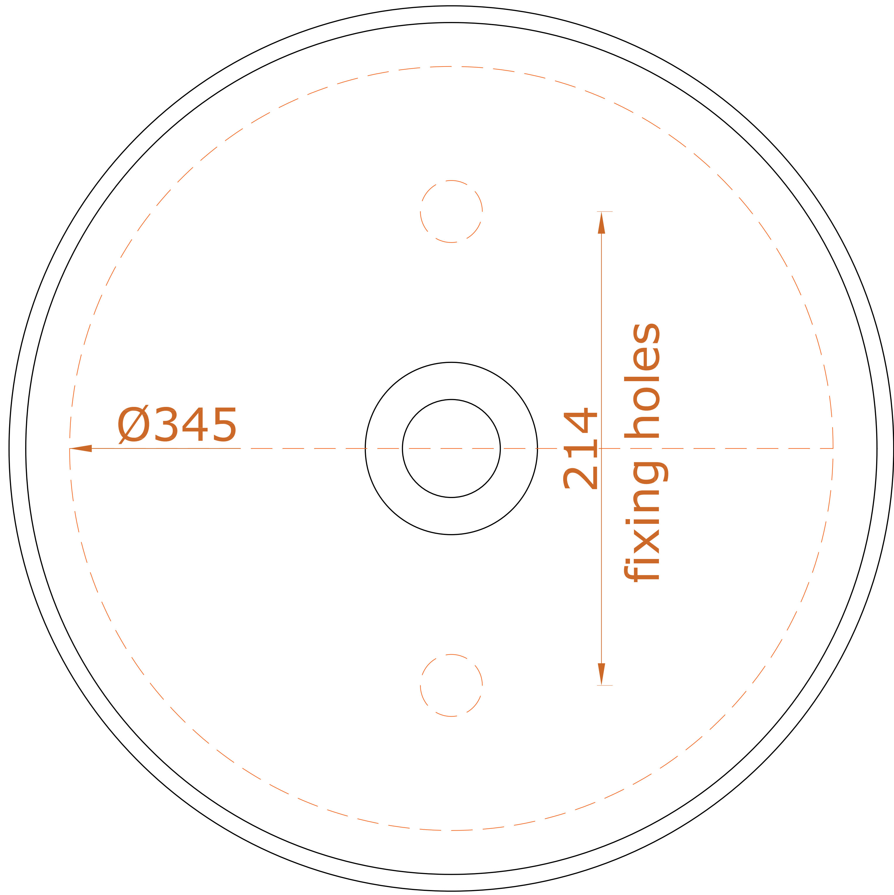
dima incasso
