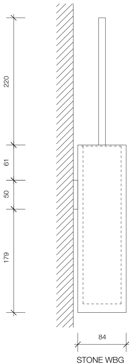
Seitenansicht Side view
