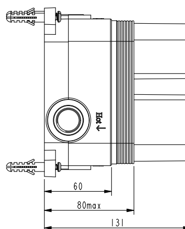
Габаритные размеры
