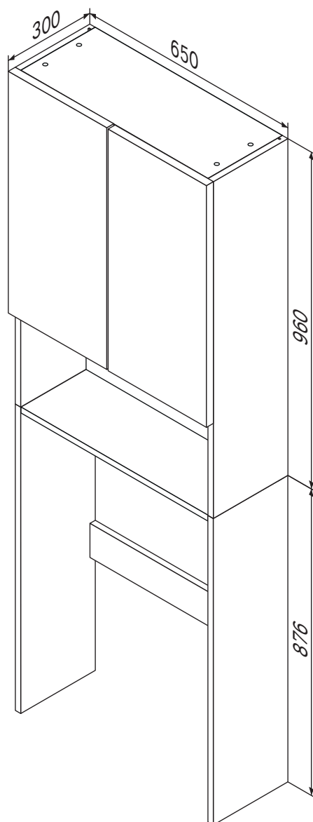
X-Joy M85CSX06521WG1
