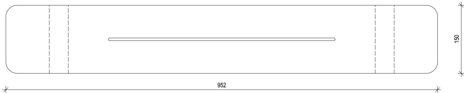
Draufsicht Top view
